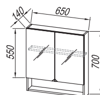
TOE 65
