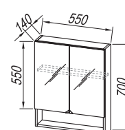
TOE 55
