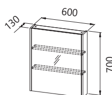
TOB 60
