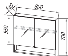
TOE 80
