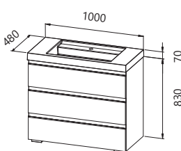
OUHF 100 CO OUHF 100 LG OUHF 100 BO
