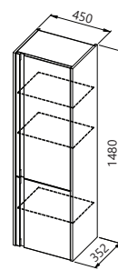
J 1482/450 LG J 1482/450 CR J 1482/450 BO
