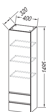
OUN 70 WH OUN 70 NW OUN 70 DC
