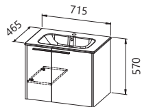
OUB 70 WH OUB 70 CM
