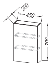
V 702/20 WH - white V 702/20 BE - beige V 702/20 DG - dark grey
