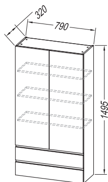
OUN 80 WH OUN 80 NW OUN 80 DC
