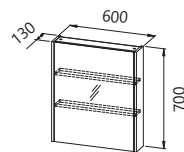
TOB 60 WH TOB 60 CM
