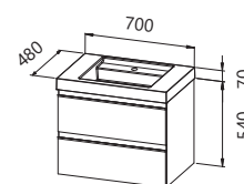
OUHW 70 CO OUHW 70 LG OUHW 70 BO
